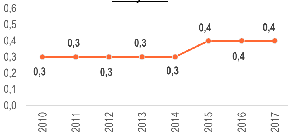
Толуолы
