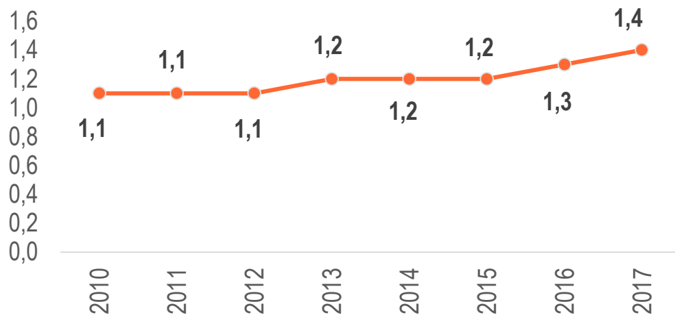
Толуолы
