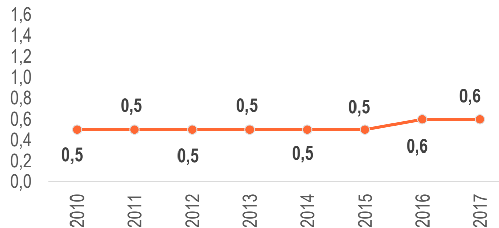
Ксилолы
